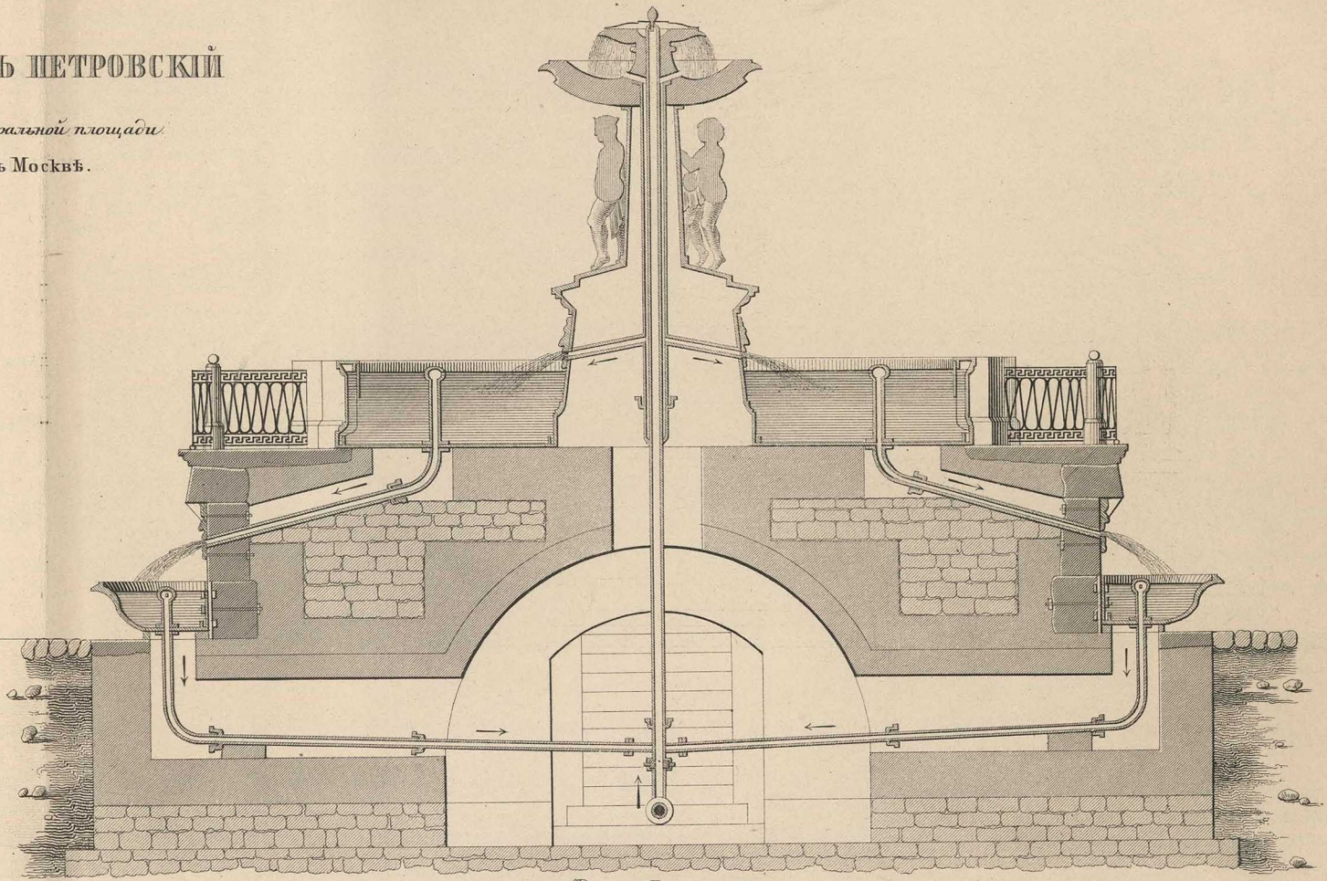
РАЗРѢЗЫ
